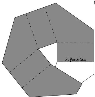
炭素原子
