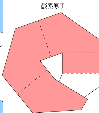
酸素原子
